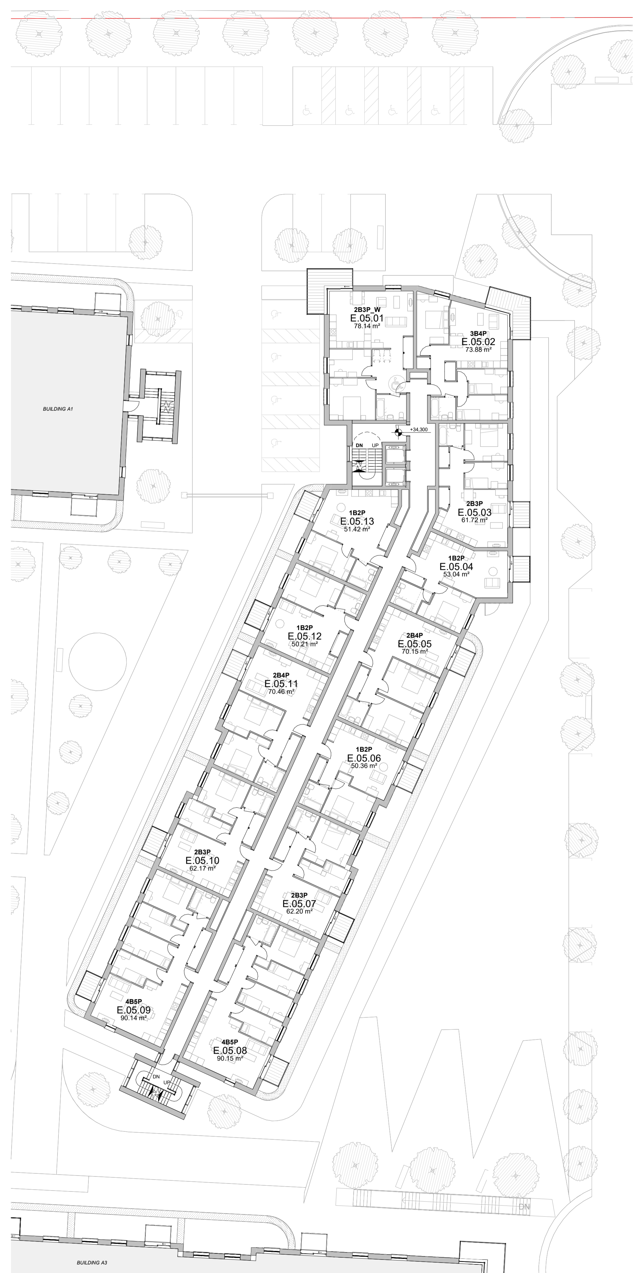
2 Level 5 +34.300 AOD 1:200
